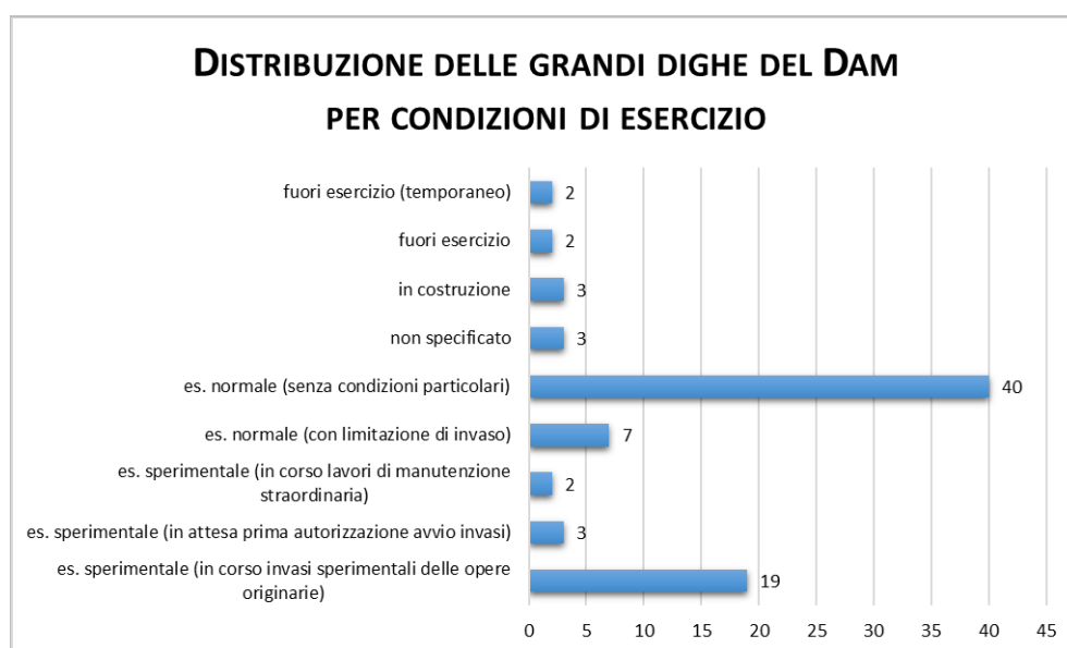
Figura 70. Distribuzione delle grandi dighe del DAM per condizioni di esercizio
