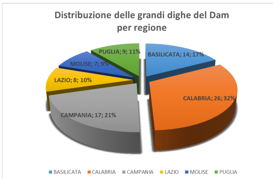
Figura 66. Distribuzione delle grandi dighe del DAM per Regione
