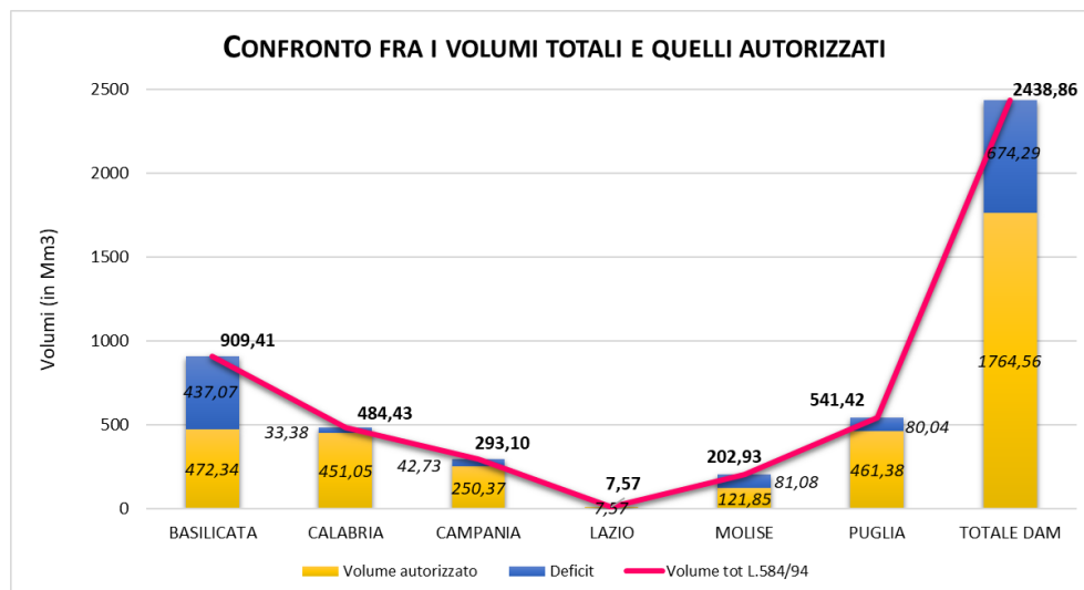
Figura 67. Confronto fra i volumi totali e quelli autorizzati delle grandi dighe delle regioni nell'ambito del DAM
