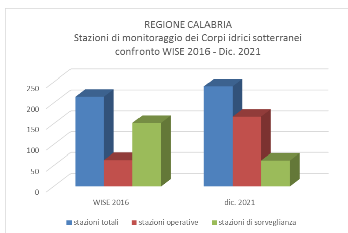
Figura 31. Stazioni di monitoraggio chimico distinte per operativo e sorveglianza riportate nel WISE 2016 e l'aggiornamento a Dicembre 2021.
