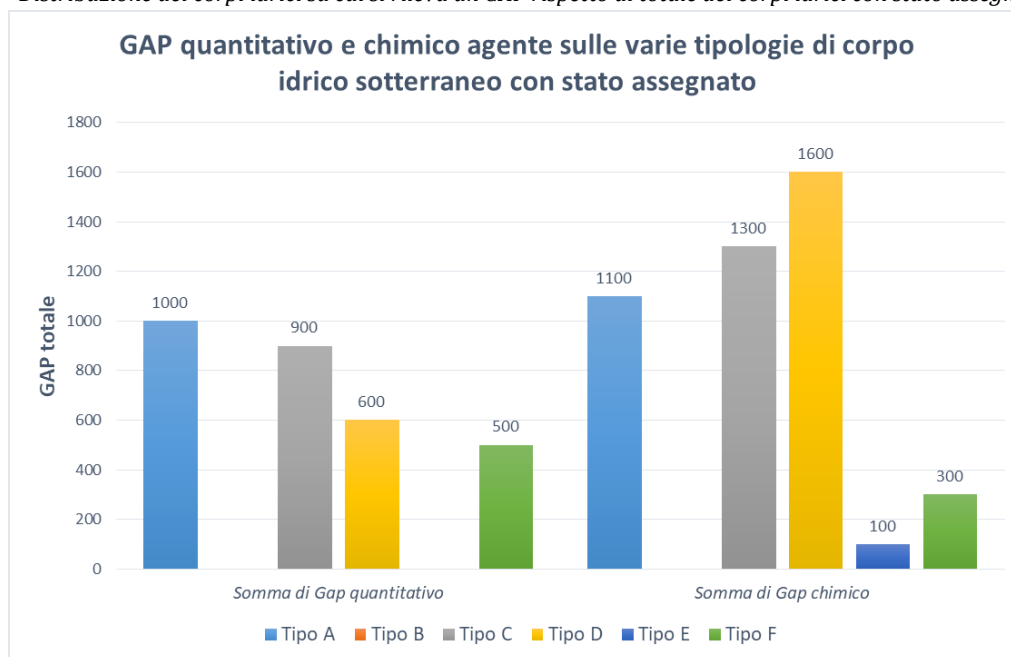
Figura 58 - Distribuzione del GAP (in termini assoluti) chimico e quantitativo per tipologia di corpi idrici con stato assegnato.
