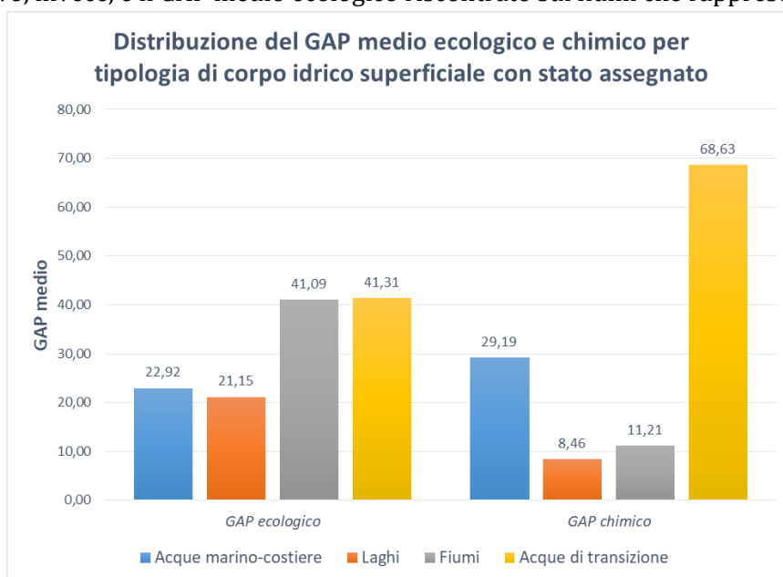
Figura 56 - Distribuzione del GAP medio chimico ed ecologico per tipologia di corpi idrici con stato assegnato.
