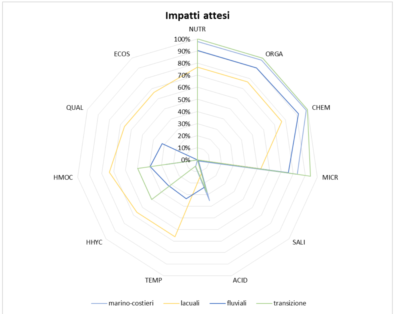
Figura 53. Distribuzione degli impatti attesi per le acque superficiali nel DAM.
